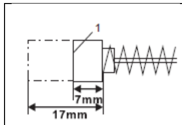
1. Отметка износа
